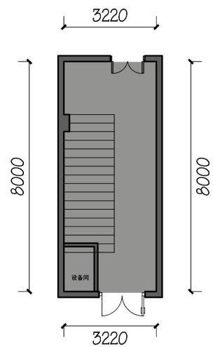
一层平面图 1:150
