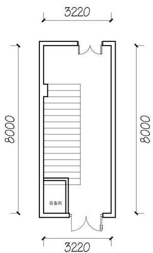
一层平面图 1:150
