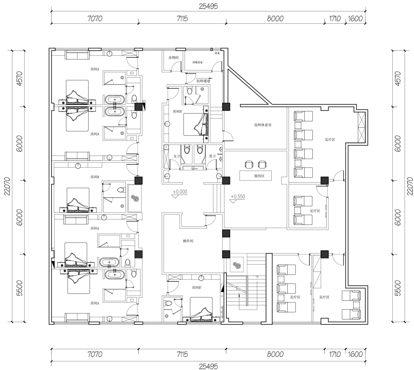
二层平面图 1:150
